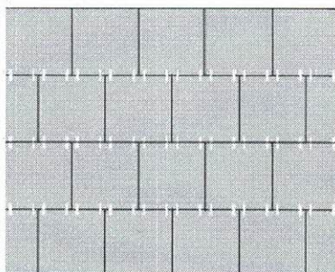
Poprawne: ułożenie "T"
