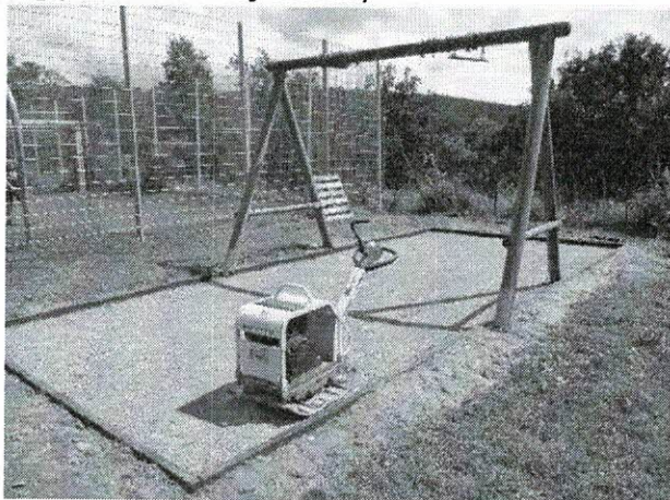
Zagęszczenie górnej warstwy
